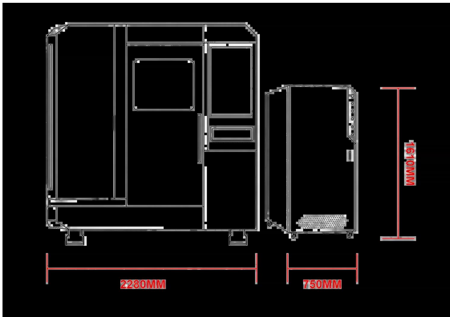
Disegno quotato della macchina Vista laterale e dall'alto con le dimensioni principali della struttura DH-1520.
