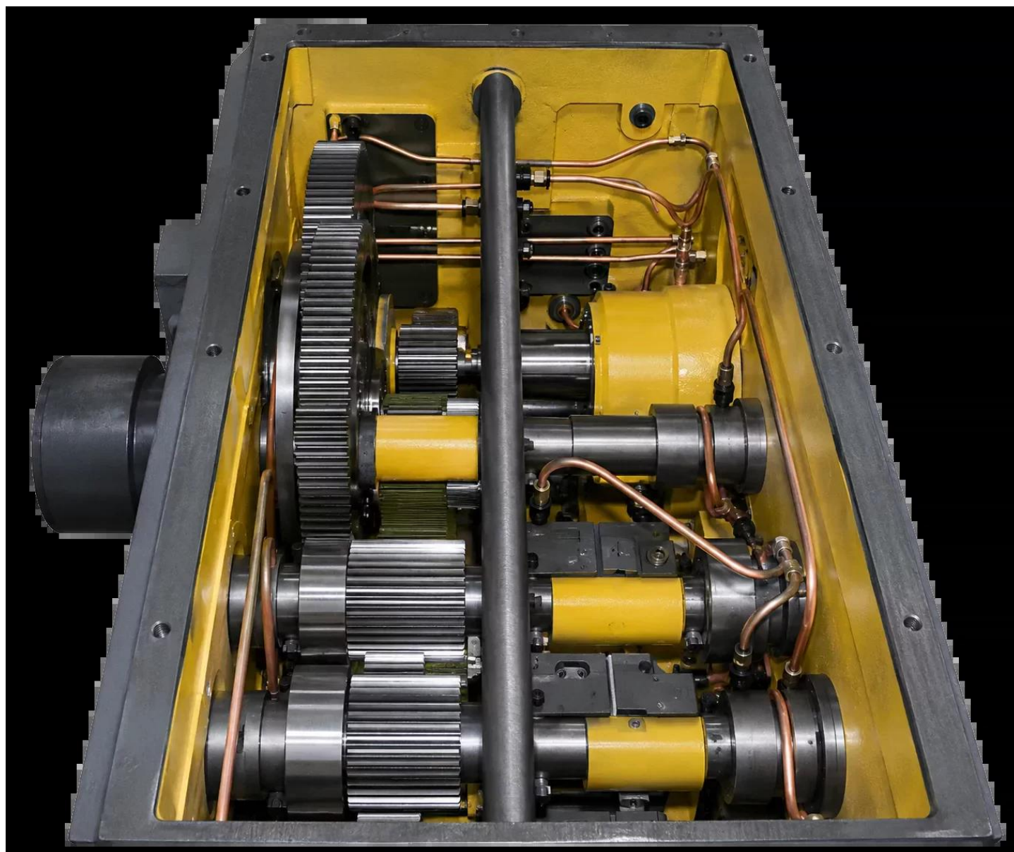
Traverse / Führungen
